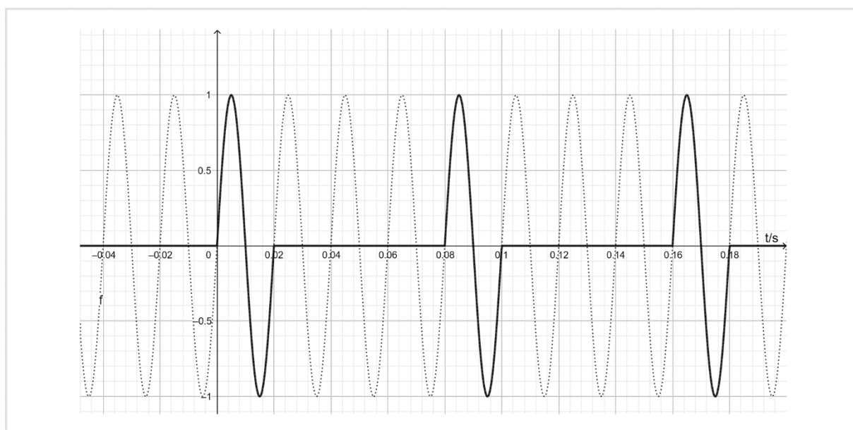
Abbildung 1 Schwingungspaketsteuerung 25 % (selbst erstellt, kann beliebig gefärbt, skaliert, umgestaltet werden)
