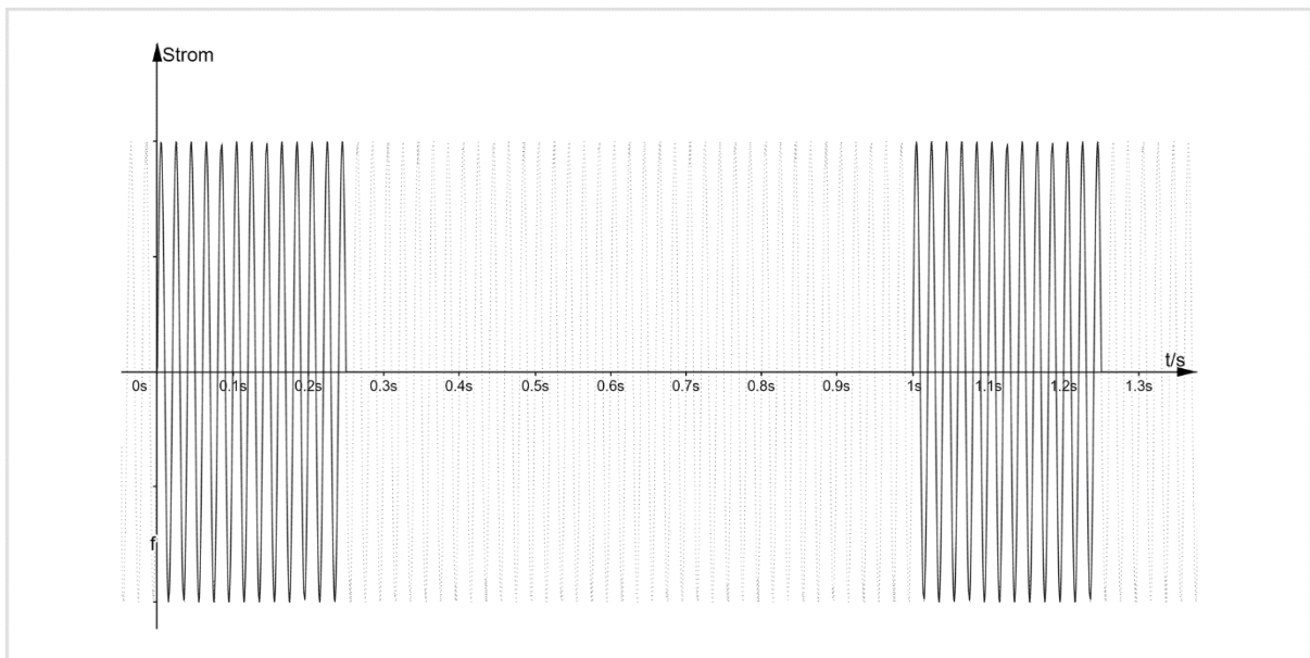
Abbildung 2 - größere Schwingungspakete
