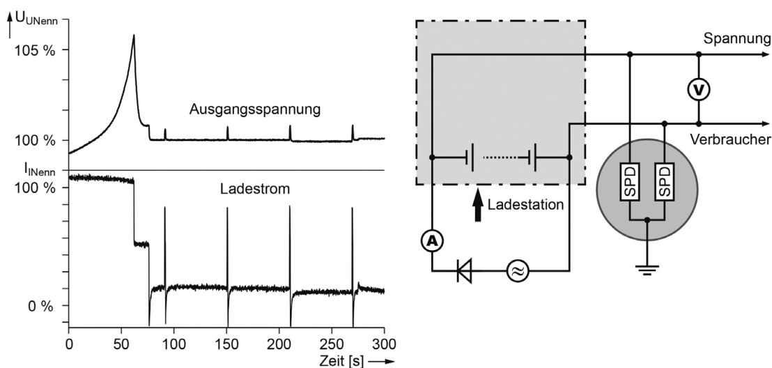
Abbildung 3 – Starkladung batteriegespeicherter Stromversorgungen [19]
