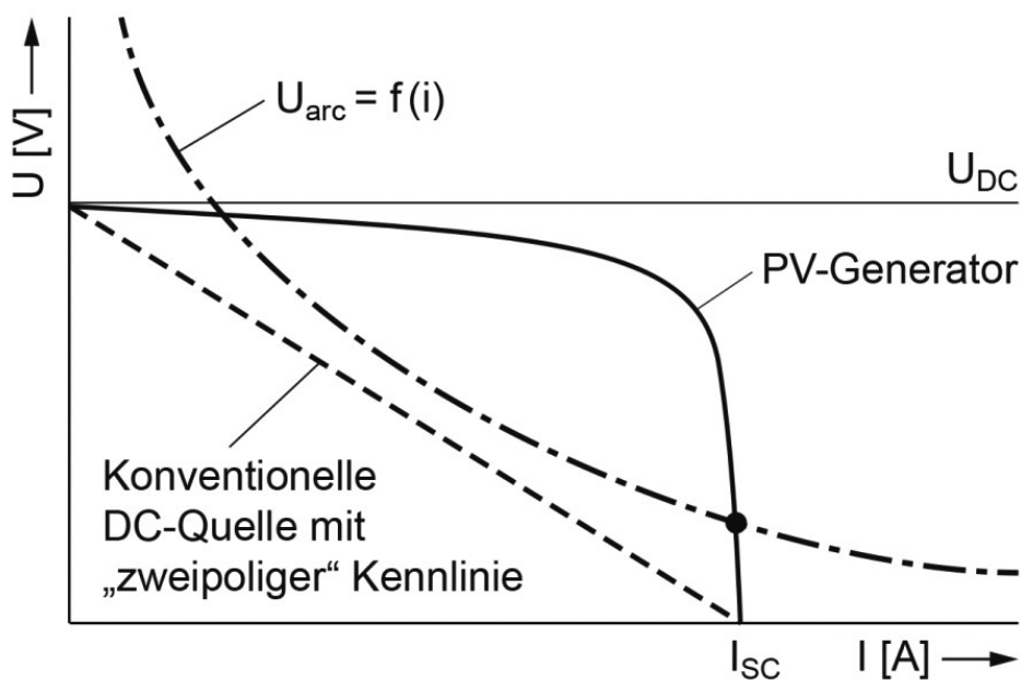
Abbildung 11 – PV-Quelle und konventionelle DC-Quelle [19]
