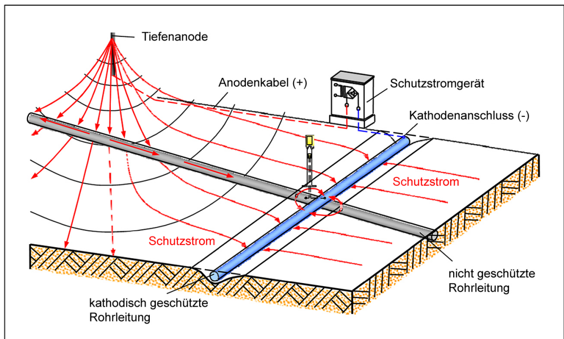
Abbildung 7 – Spannungsverlauf einer Anodenanlage einer geschützten Rohrleitung
