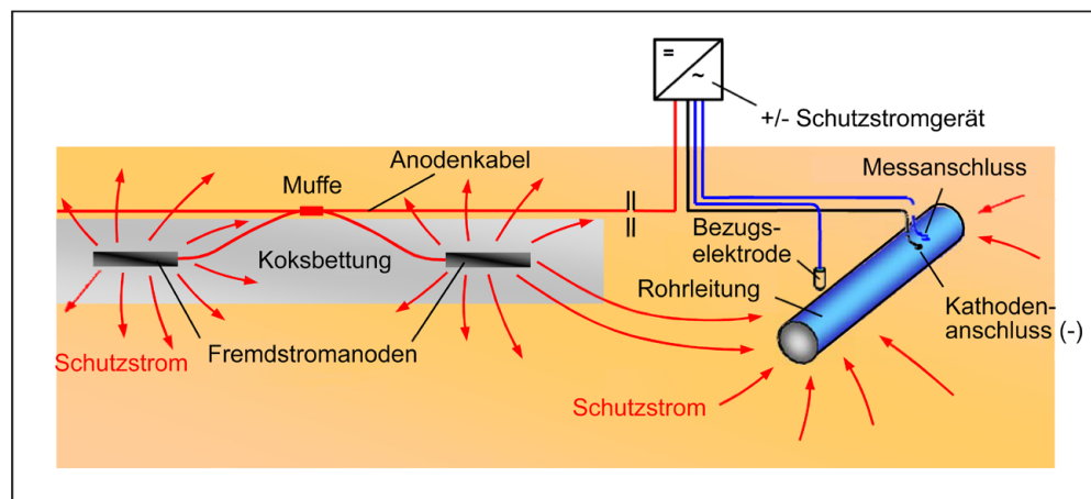
Abbildung 8 – Schutzstrom
